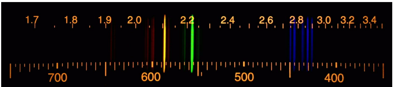
Krypton (Kr)
