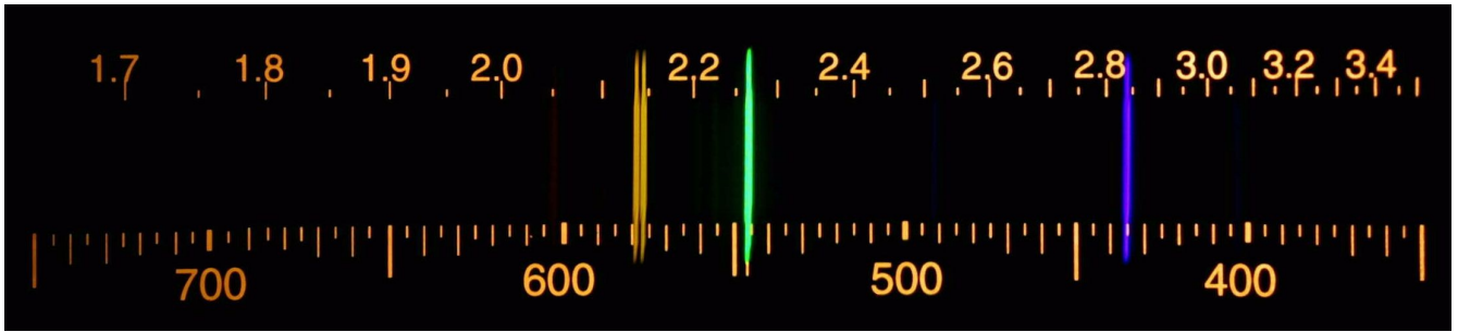
Mercury (Hg)
