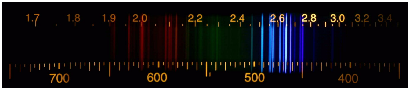
Xenon (Xe)
